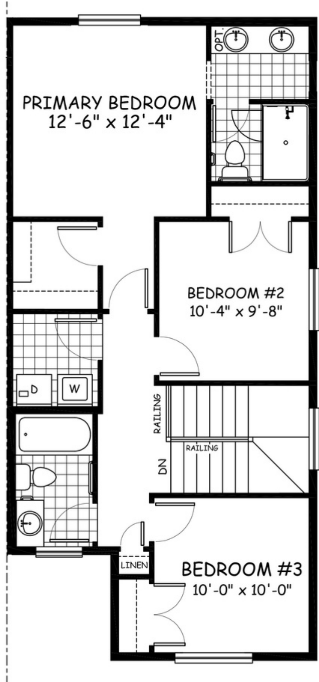
UPPER 722 sq.ft.
